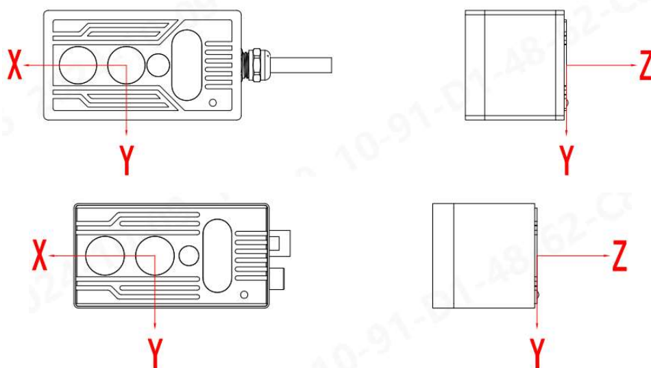
图 4.4 相机原点示意图
