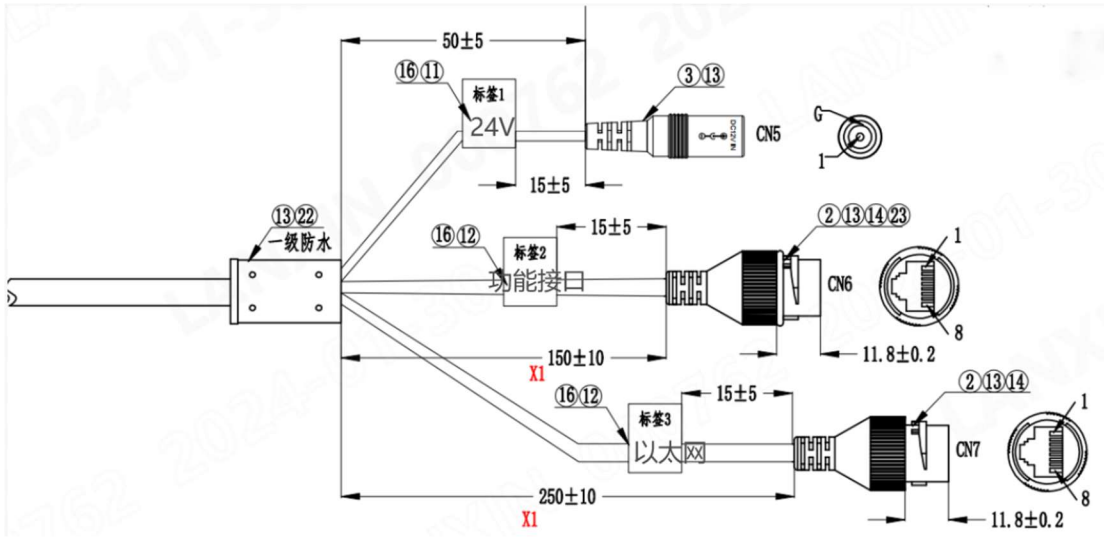
图 2.1 引脚说明
