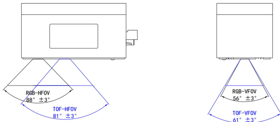
图 4.2 M4 视场范围
