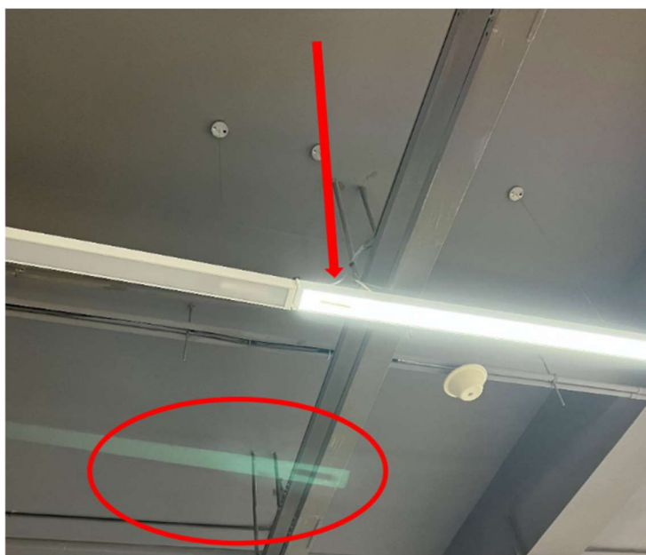
图 4.9 杂光影响 ghost 与 flare
