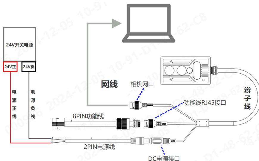
图 5.3 M4Mega 相机连接示意图
