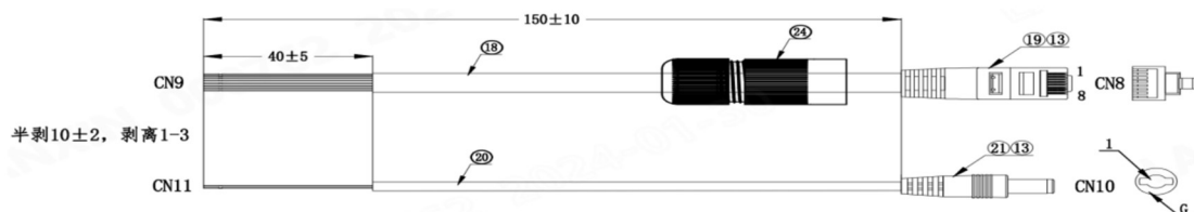
图 2.2 功能线线序说明
