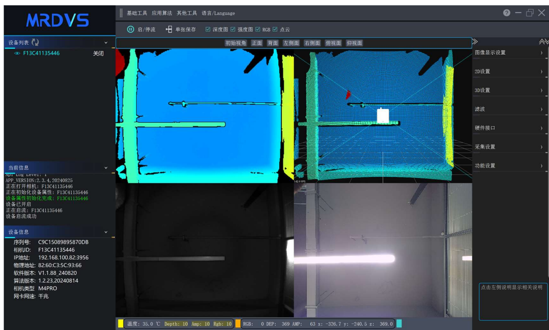
图 4.12 图像显示
