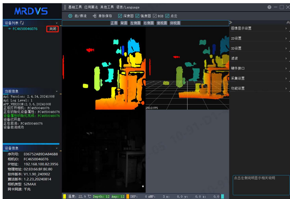
图 5.8 图像显示
