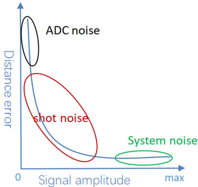
图 4.17 测量精度与信号强度关系图
