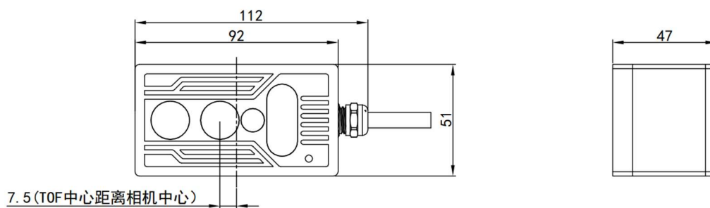
图 3.2 M4Mega 结构图纸
