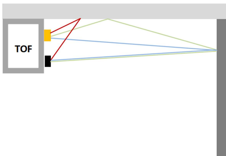
图 4.16 相机安装图
