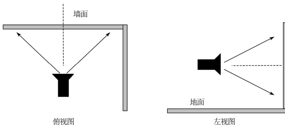
图 4.5 安装方式一
