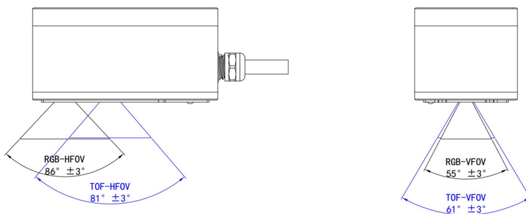
图 4.1 M4Mega 视场范围
