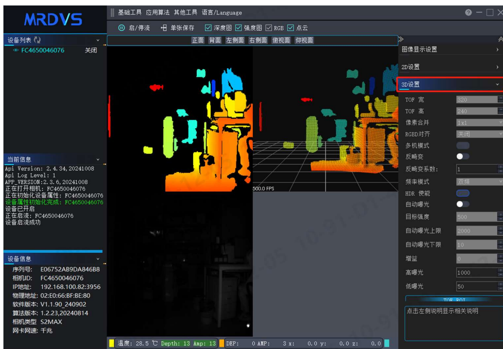
图 5.9 参数设置
