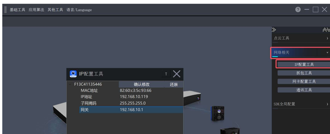
图 4.14 修改 IP
