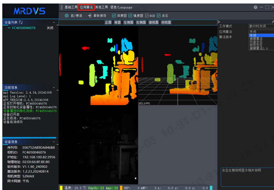
图 5.10 算法切换
