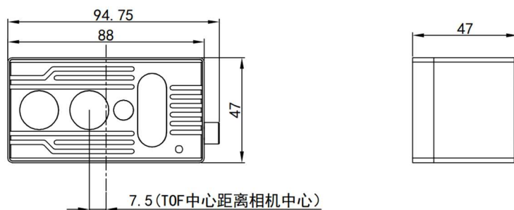
图 3.3 M4 结构图纸
