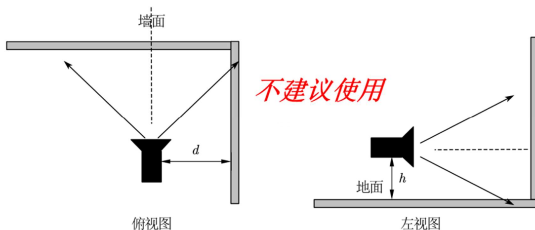
图 4.10 不建议使用的安装方式
